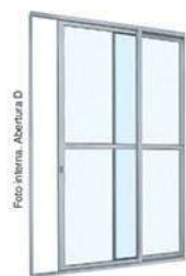
PCC 2F Porta de Correr com Divisão Central - 2 folhas 216x160x6,6 - 2 • D 78.50.603-2 216x160x6,6 - 2 • E 78.50.604-0 Vidro Liso Vidro Temperado abaixo de 1,10m de altura.*
