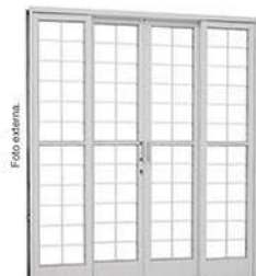
PCQ 4F Porta de Correr com Grade Quadriculada - 4 folhas 217x200x12 - 4 • 26.32.450-5 Vidro Temperado abaixo de 1,10m de altura.*
